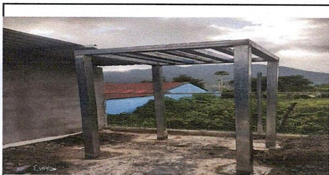
Foto 5: HECHA E INSTLACIÓN DE BASE DE ESTRUCTURA METÁLICA PARA ROTOPLAS.
